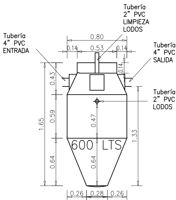
DETALLE BIO – A 600 LTS ESC. 1:30
