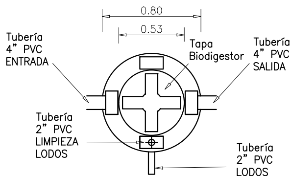
VISTA SUPERIOR ESC. 1:30
