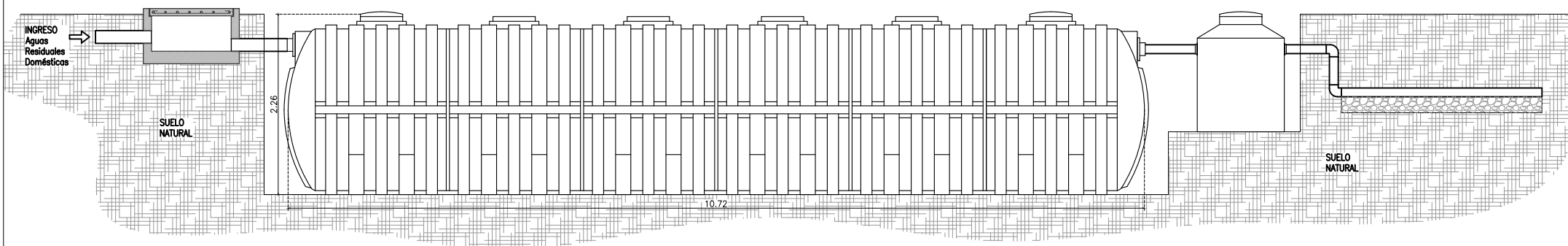
SECCIÓN LONGITUDINAL - BIODIGESTOR 30000L
