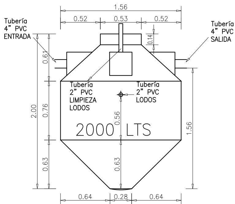
DETALLE BIO – A 2000 LTS ESC. 1:30
