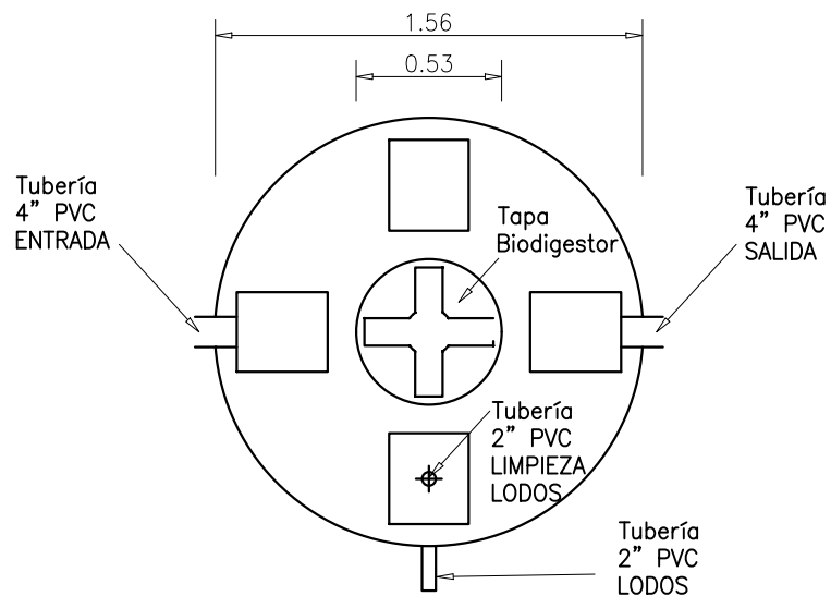
VISTA SUPERIOR ESC. 1:30
