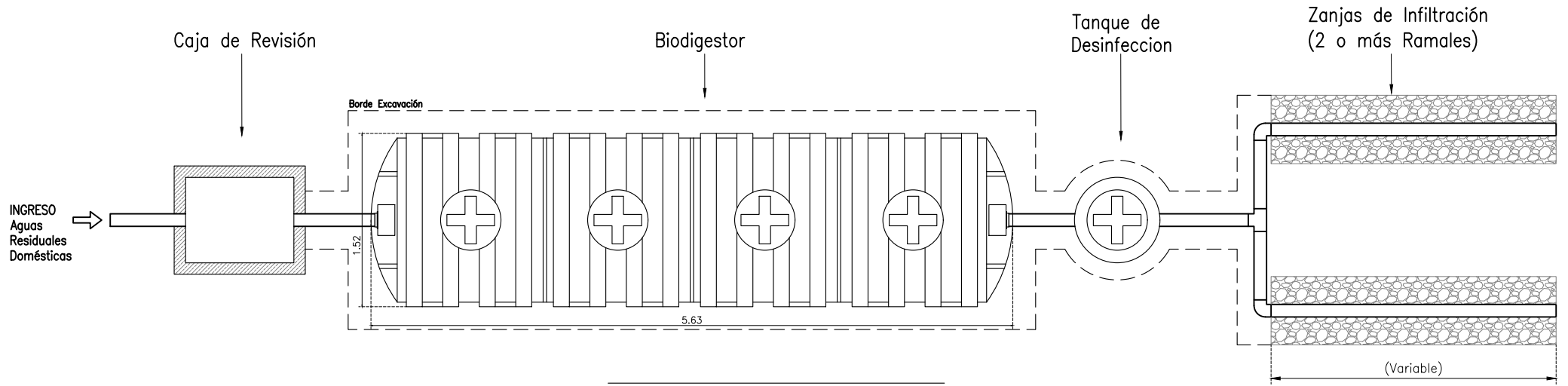
IMPLANTACIÓN GENERAL - BIODIGESTOR 10000L
