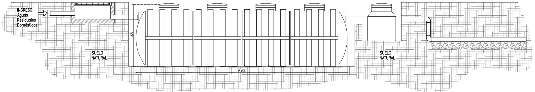
SECCIÓN LONGITUDINAL - BIODIGESTOR 10000L
