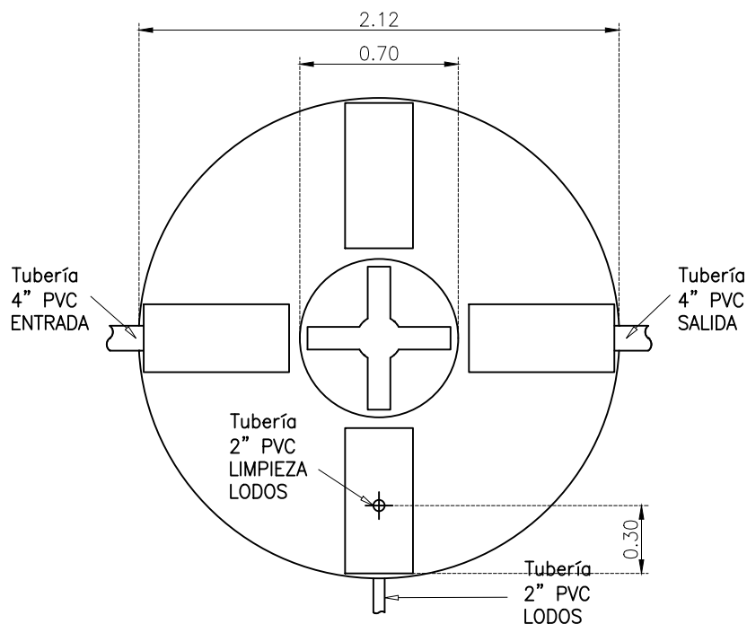
VISTA SUPERIOR ESC. 1:30
