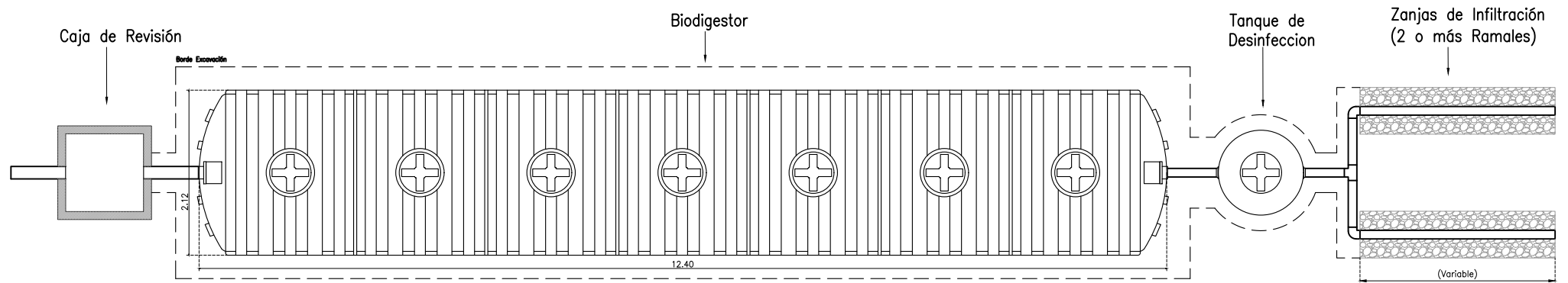
IMPLANTACIÓN GENERAL - BIODIGESTOR 35000L
