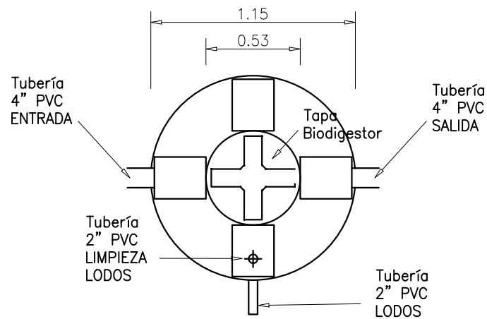
VISTA SUPERIOR ESC. 1:30
