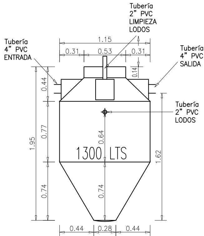
DETALLE BIO – A 1300 LTS ESC. 1:30
