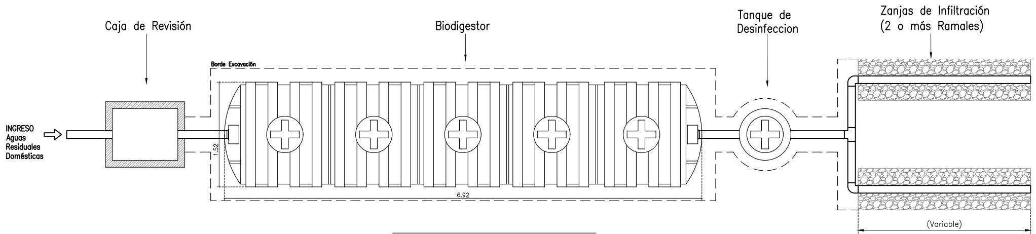
IMPLANTACIÓN GENERAL - BIODIGESTOR 12500L
