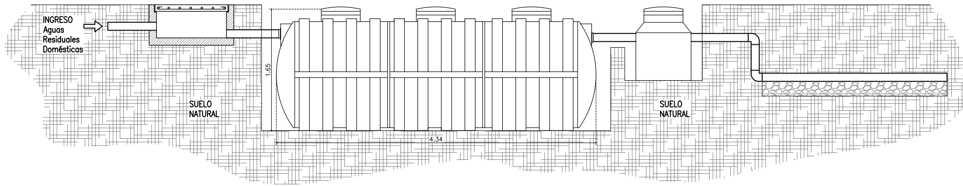
SECCIÓN LONGITUDINAL - BIODIGESTOR 7500L
