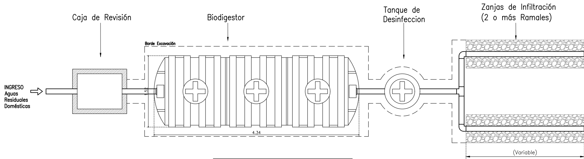
IMPLANTACIÓN GENERAL - BIODIGESTOR 7500L
