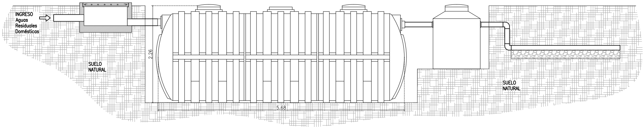
SECCIÓN LONGITUDINAL - BIODIGESTOR 15000L
