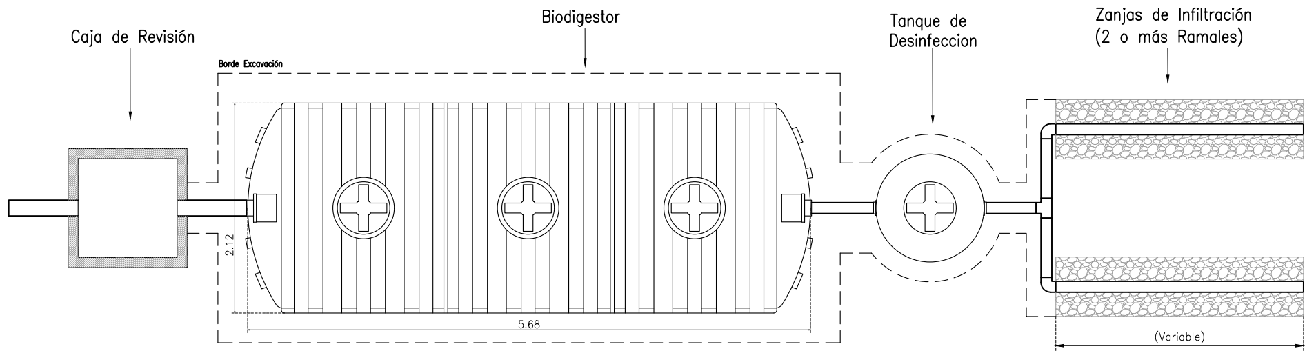
IMPLANTACIÓN GENERAL - BIODIGESTOR 15000L
