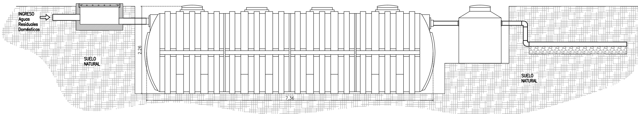
SECCIÓN LONGITUDINAL - BIODIGESTOR 20000L
