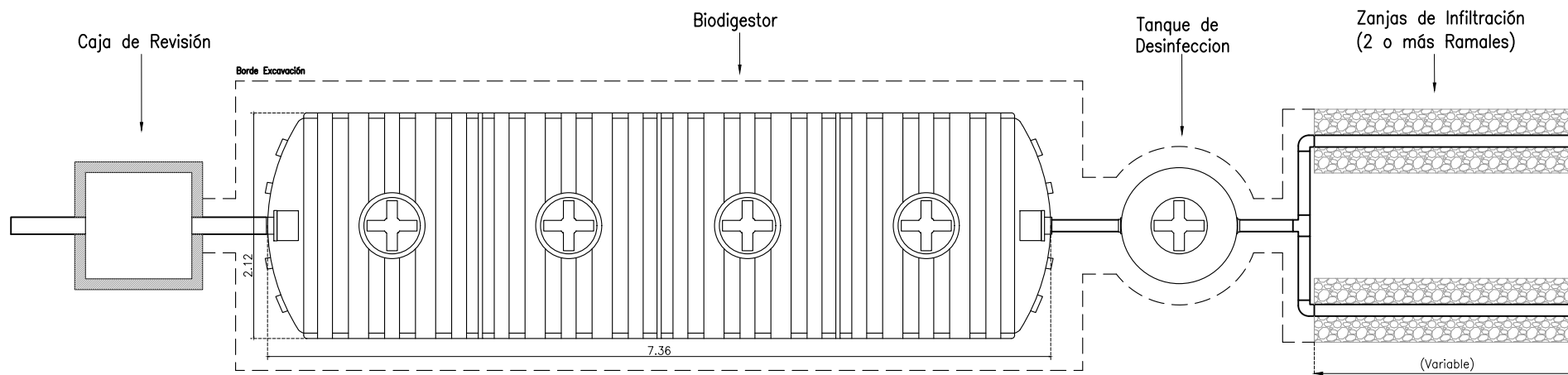
IMPLANTACIÓN GENERAL - BIODIGESTOR 20000L
