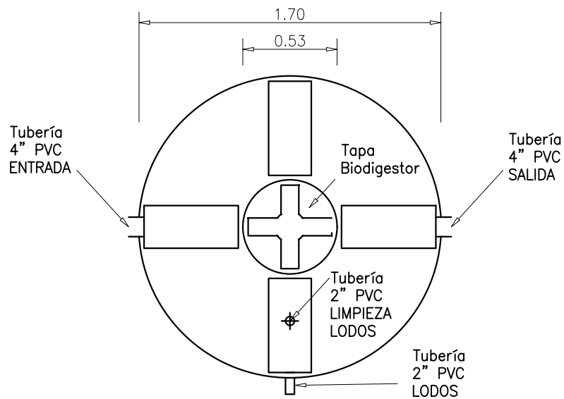
VISTA SUPERIOR ESC. 1:30
