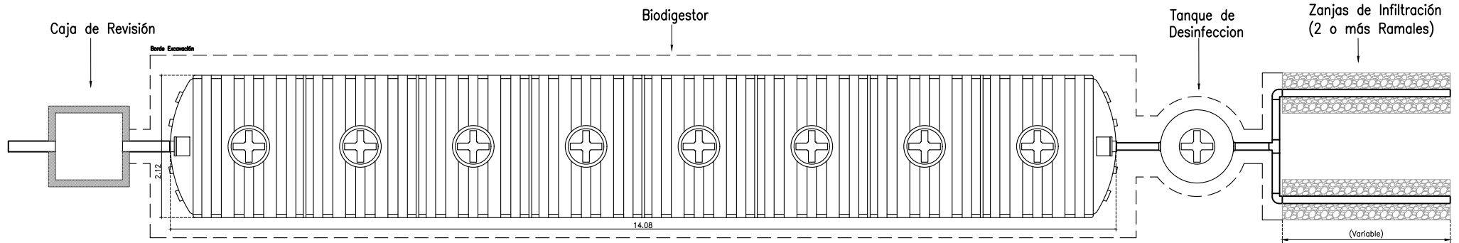
IMPLANTACIÓN GENERAL - BIODIGESTOR 40000L
