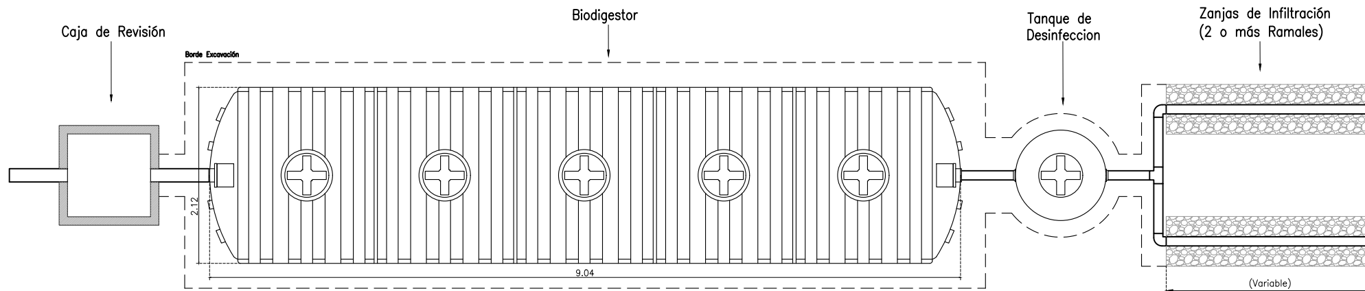
IMPLANTACIÓN GENERAL - BIODIGESTOR 25000L
