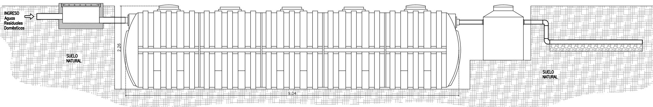
SECCIÓN LONGITUDINAL - BIODIGESTOR 25000L
