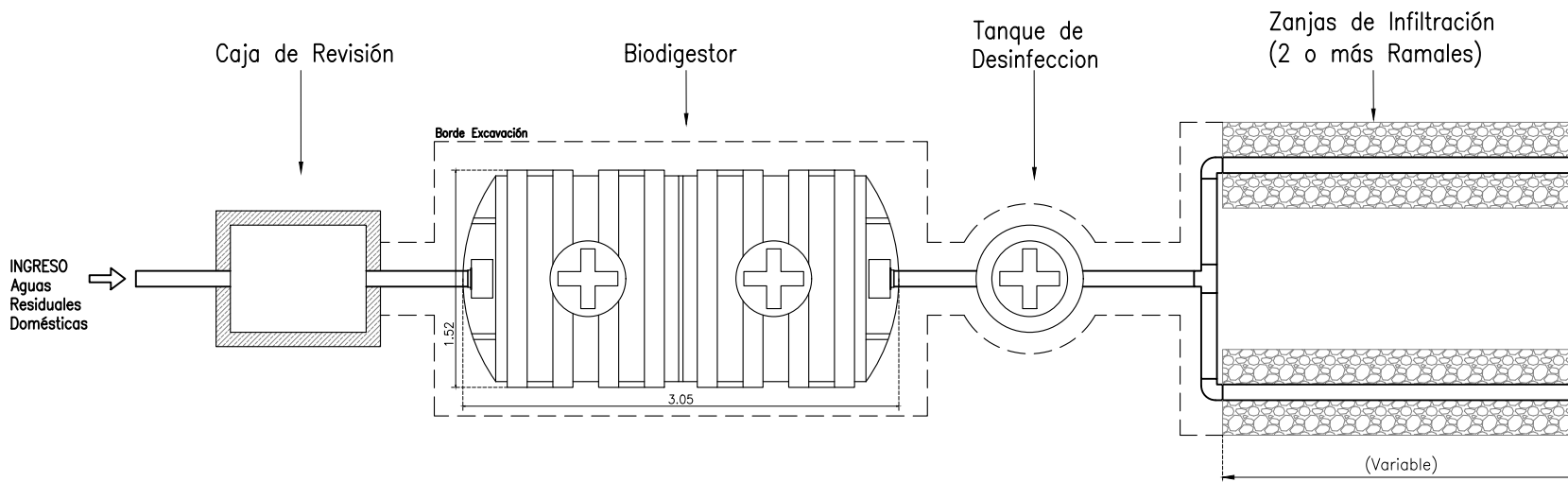
IMPLANTACIÓN GENERAL - BIODIGESTOR 5000L
