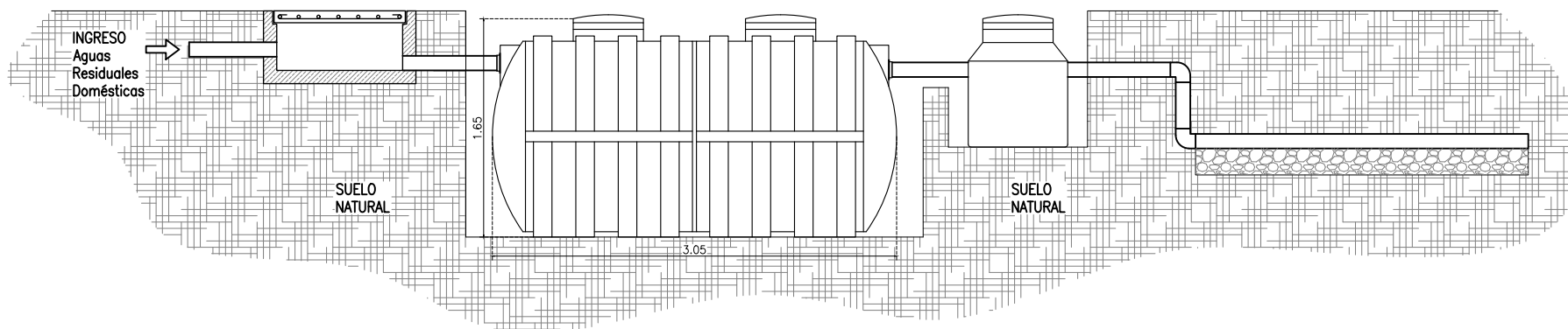
SECCIÓN LONGITUDINAL - BIODIGESTOR 5000L
